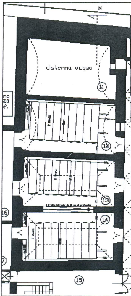
TRAPANI - Ex Convento di S. Anna - Planimetria piano terra
